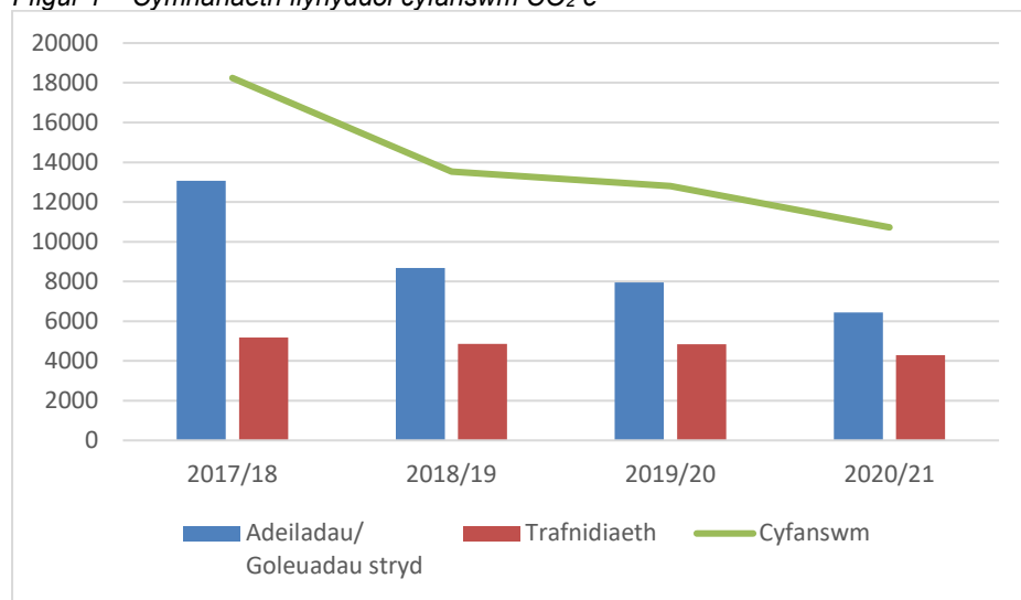
Ffigur 1 – Cymhariaeth flynyddol cyfanswm CO 2 e
